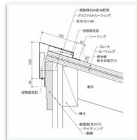
片流れ棟
