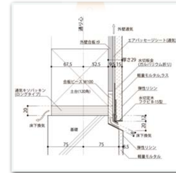
土台水切レス
