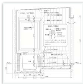
2階在来浴室
