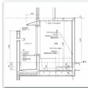
バスコートのある浴室
