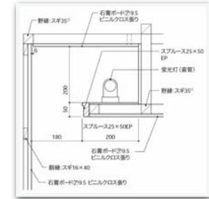
一般的な間接照明
