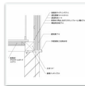
外張り断熱 - 基礎
