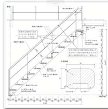
鉄骨階段 - シャープ
