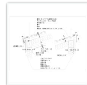
金属屋根通気
